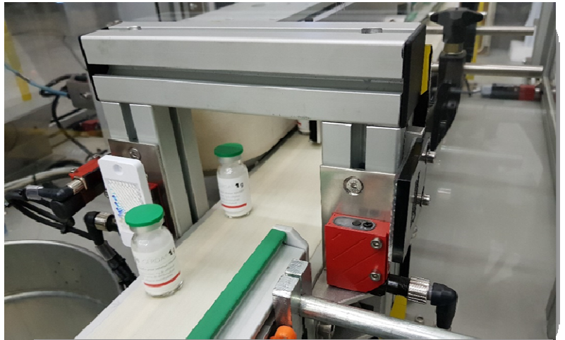
Contrôle d'application d'étiquette et impression. Label and print detection.
