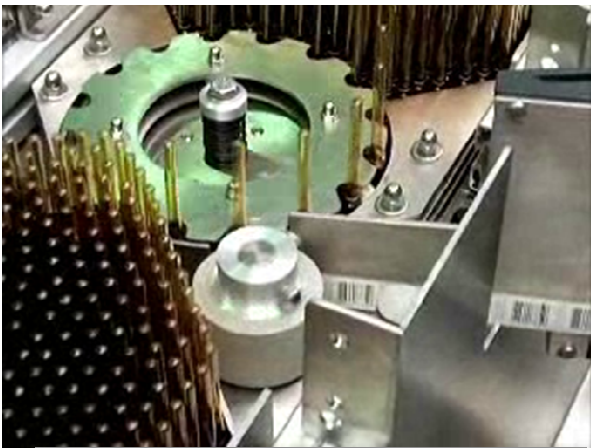
Étiquetage d'ampoules verticale et horizontale. Vertical and horizontal ampouls application.
